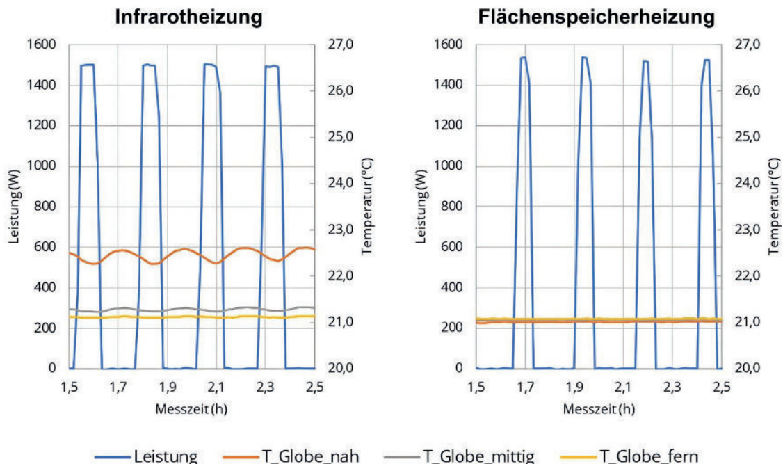
Energieverbrauch und Temperaturmessungen über Globe-Thermometer in drei verschiedenen Entfernungen zum Heizkörper
